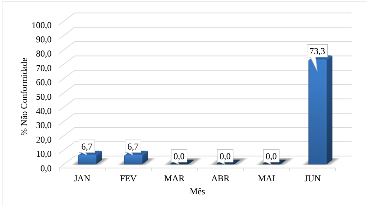
Gráfico 44 - Dados de percentual de amostras não conformes para o parâmetro Cor Aparente. Fonte: DESO, 2023.
