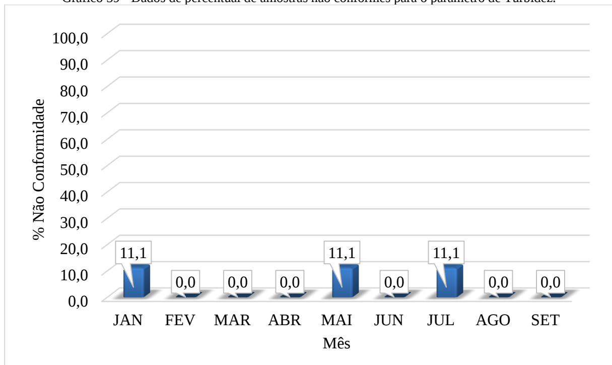
Gráfico 39 - Dados de percentual de amostras não conformes para o parâmetro de Turbidez.
