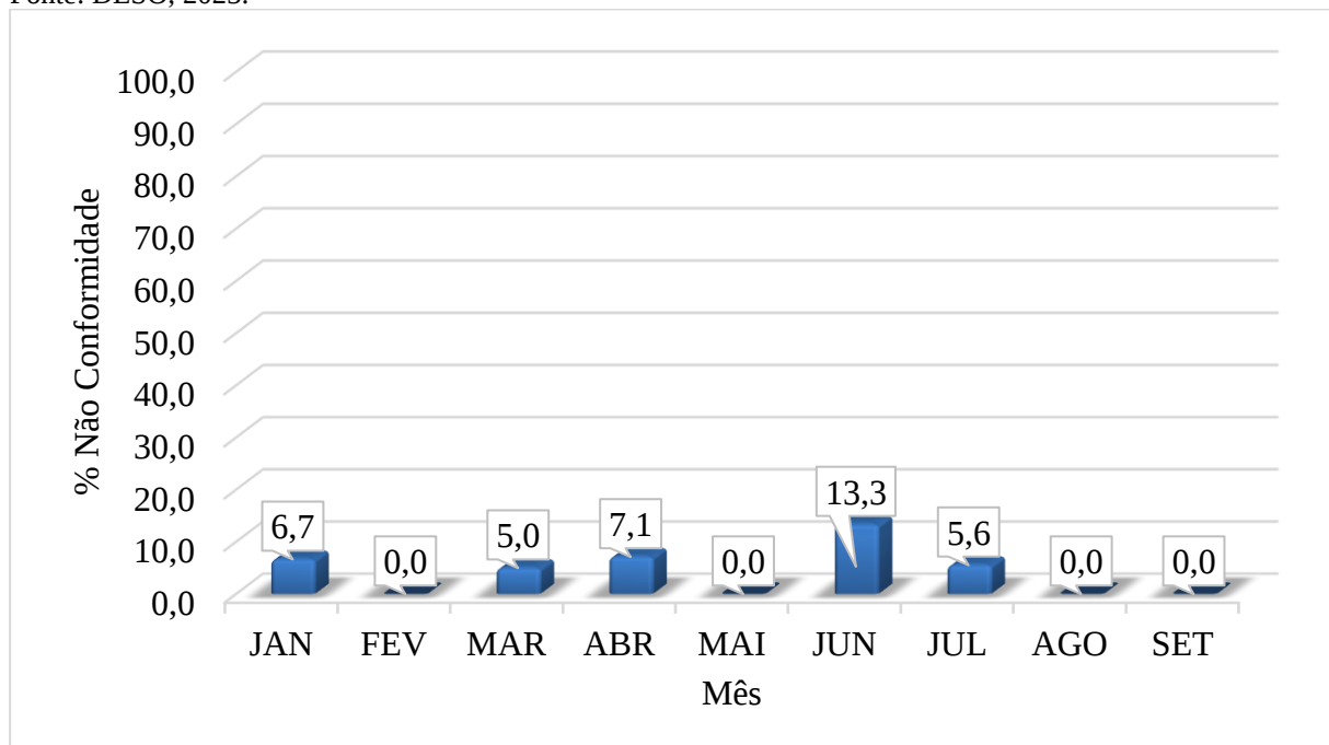
Gráfico 43 - Dados de percentual de amostras não conformes para o parâmetro de Cloro Residual Livre. Fonte: DESO, 2023.
