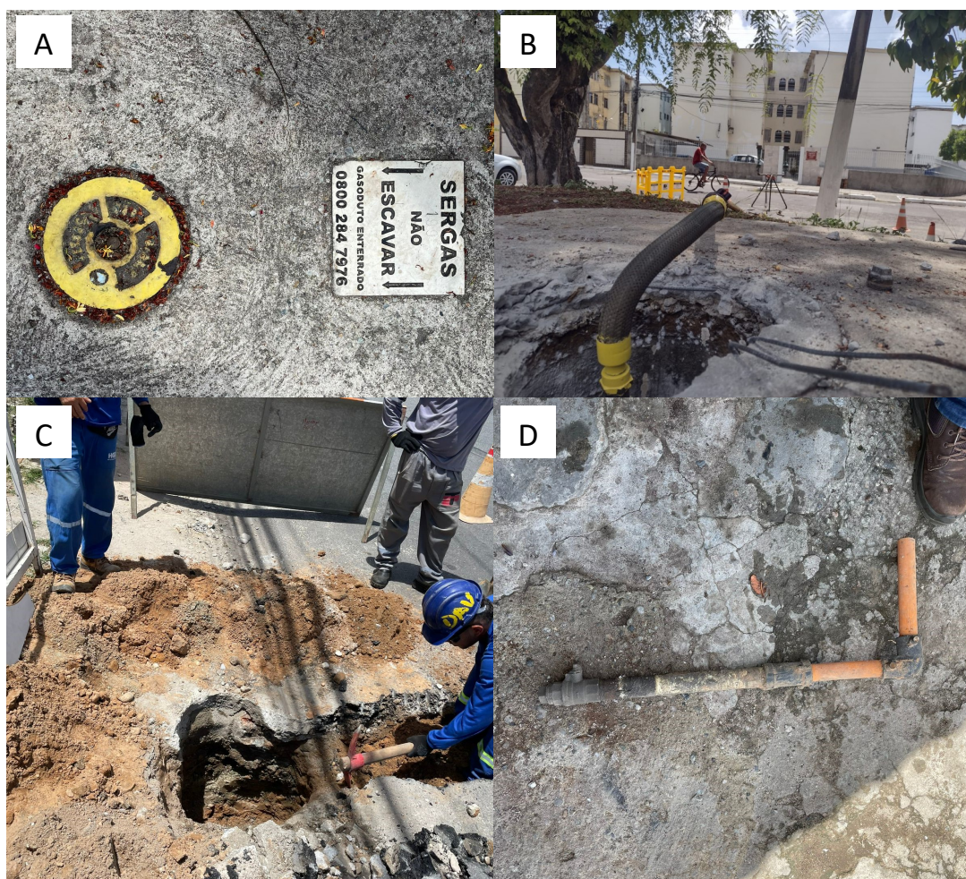
Figura 1: Manutenção Preventiva do gasoduto da Av. Rio de Janeiro
