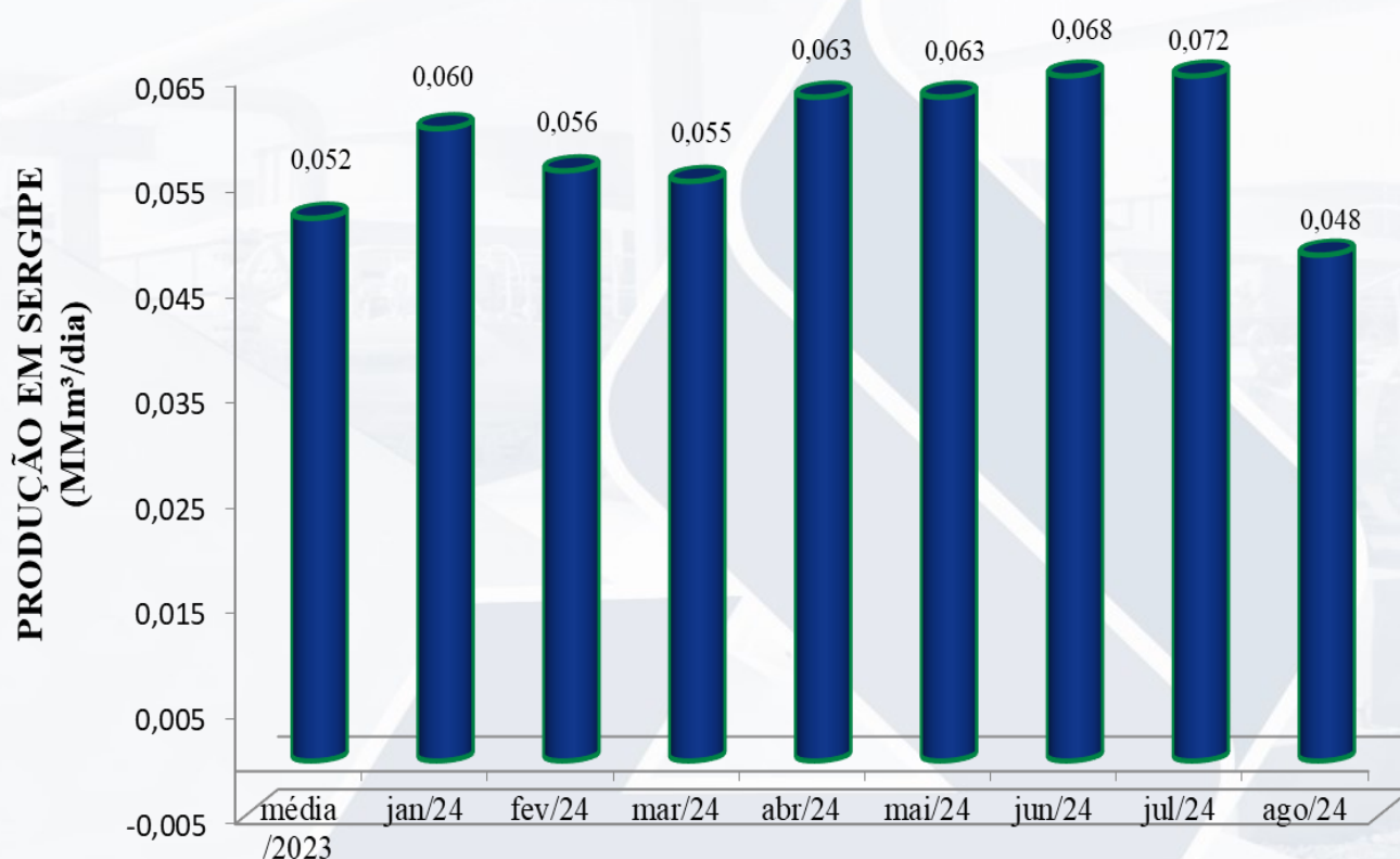
Gráfico 09: Produção de gás natural em Sergipe.
