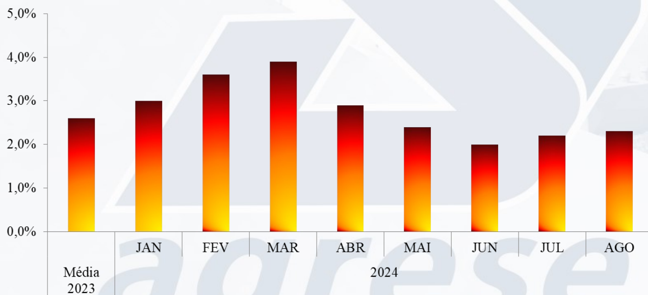
Gráfico 3: Queima de Gás Natural em Relação à Produção Nacional de Gás Natural (Agosto/2024).
