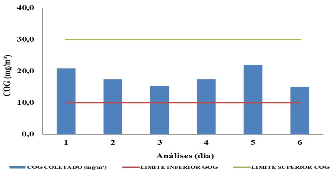
Gráfico 2: Análise Cromatográfica (COG)
