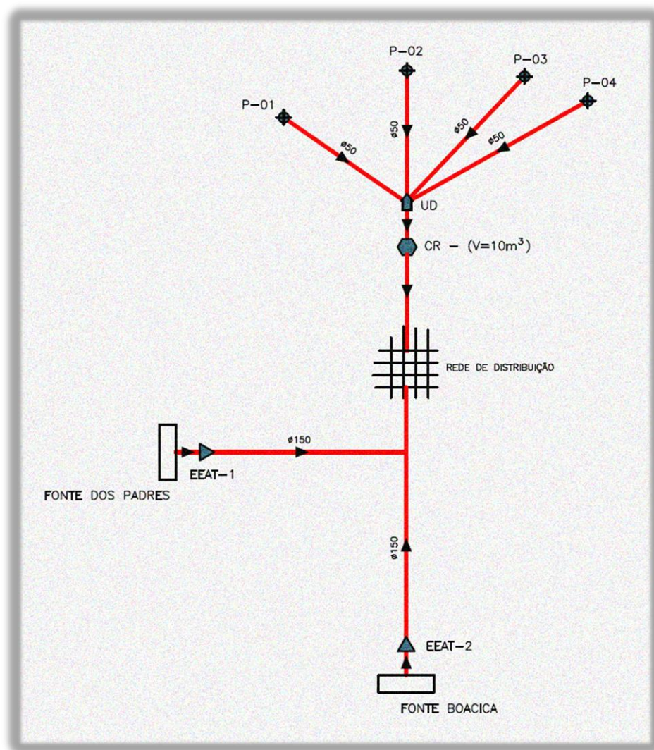
Figura 6 - Diagrama simplificado do sistema Divina Pastora – SEDE
