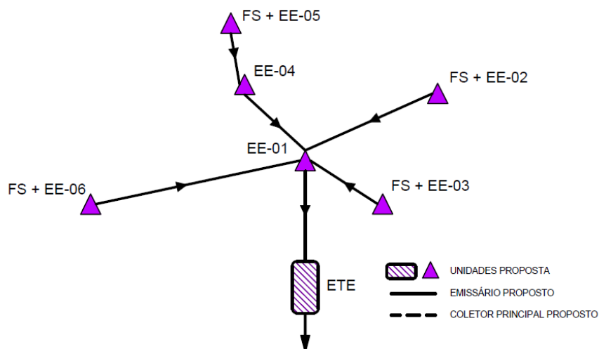
Figura 8 - Sistema de interligação das elevatórias
