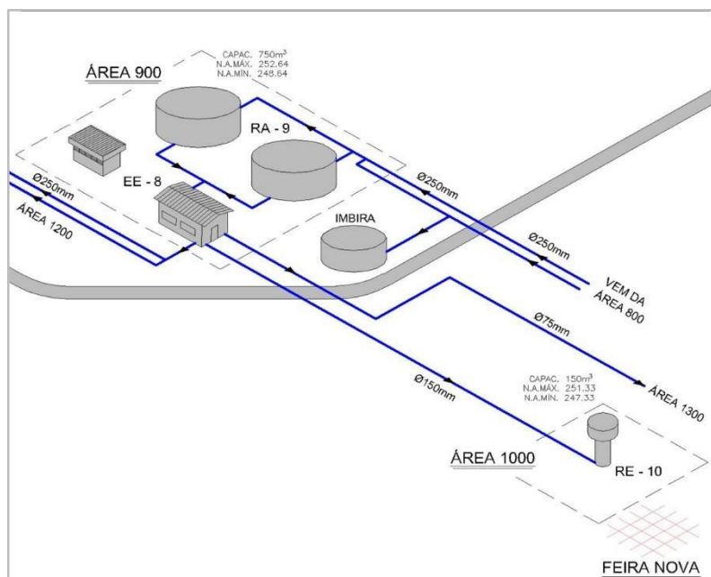
Figura 7 - Sistema de Abastecimento de Água
