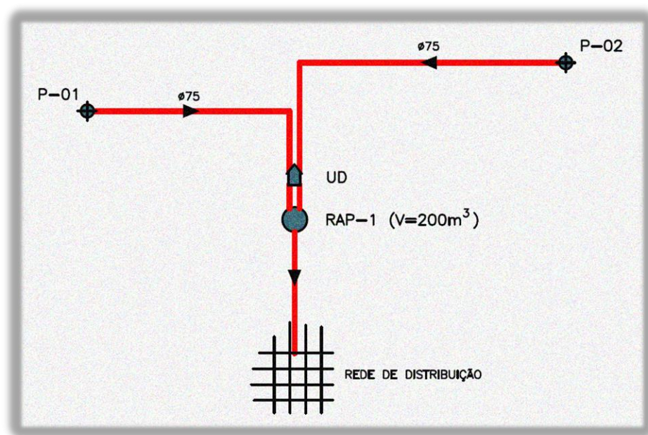
Figura 6 - Diagrama simplificado do sistema General Maynard – SEDE
