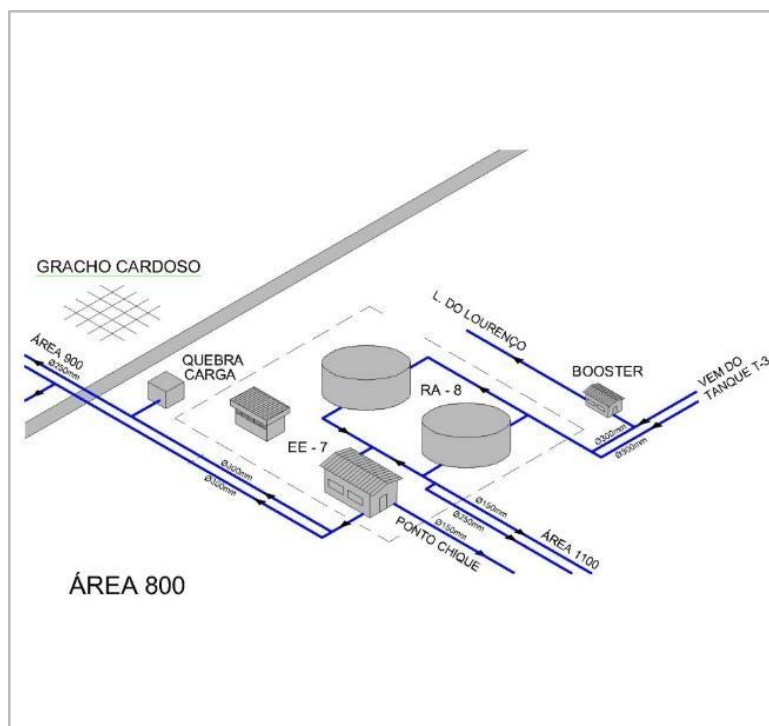
Figura 8 - Sistema de Abastecimento de Água de Graccho Cardoso
