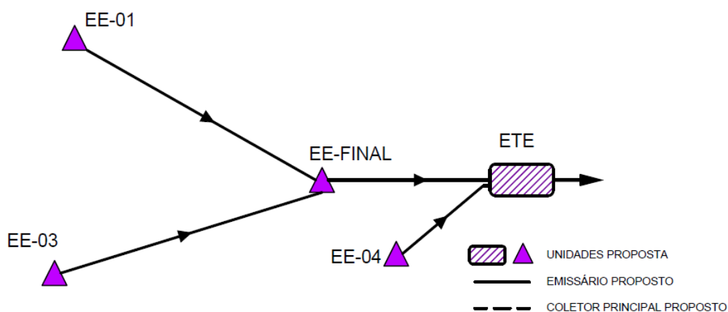
Figura 9 - Sistema de interligação das elevatórias
