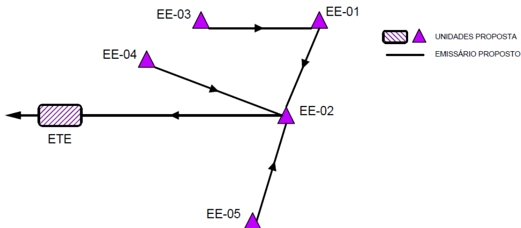
Figura 10 - Sistema de interligação das elevatórias
