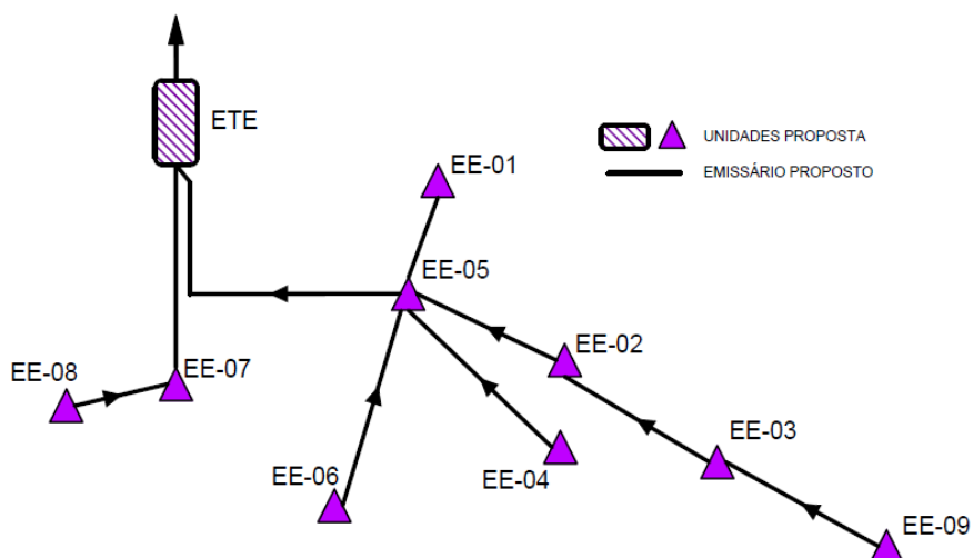
Figura 9 - Sistema de interligação das elevatórias
