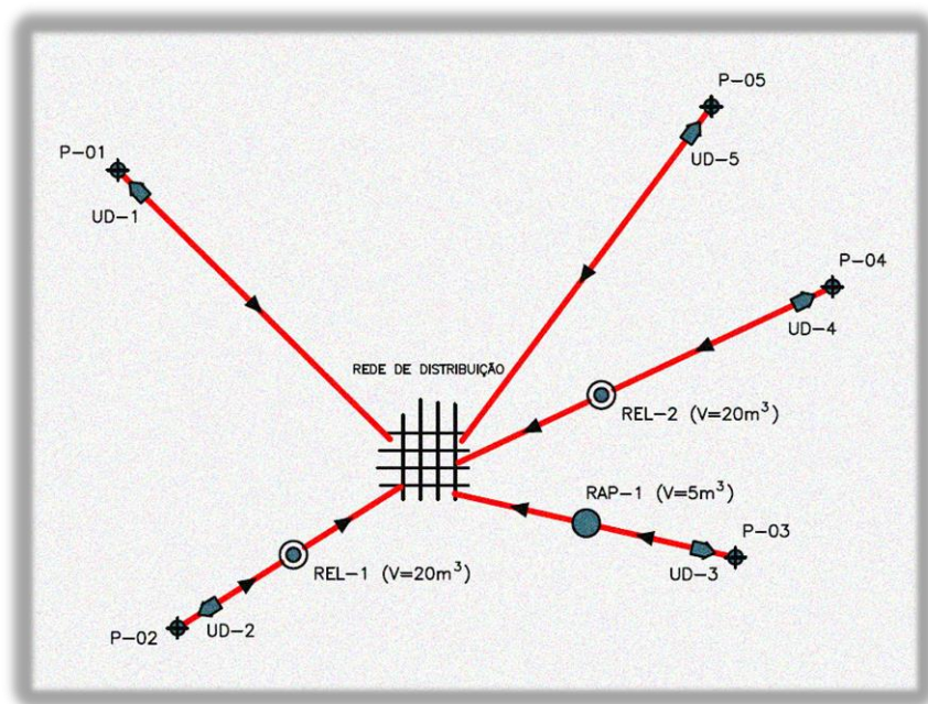
Figura 7 - Diagrama simplificado do sistema povoado Pedra Branca – Laranjeiras
