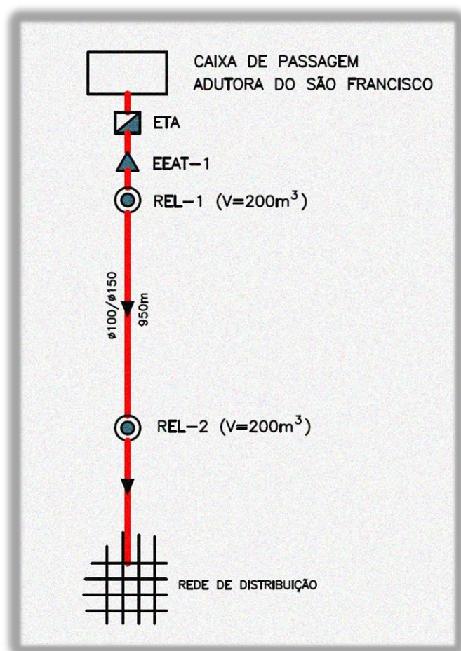
Figura 6 - Diagrama simplificado do sistema Malhada dos Bois – sede
