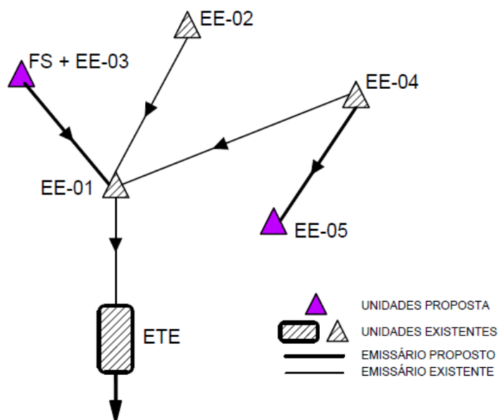
Figura 8 - Sistema de interligação das elevatórias
