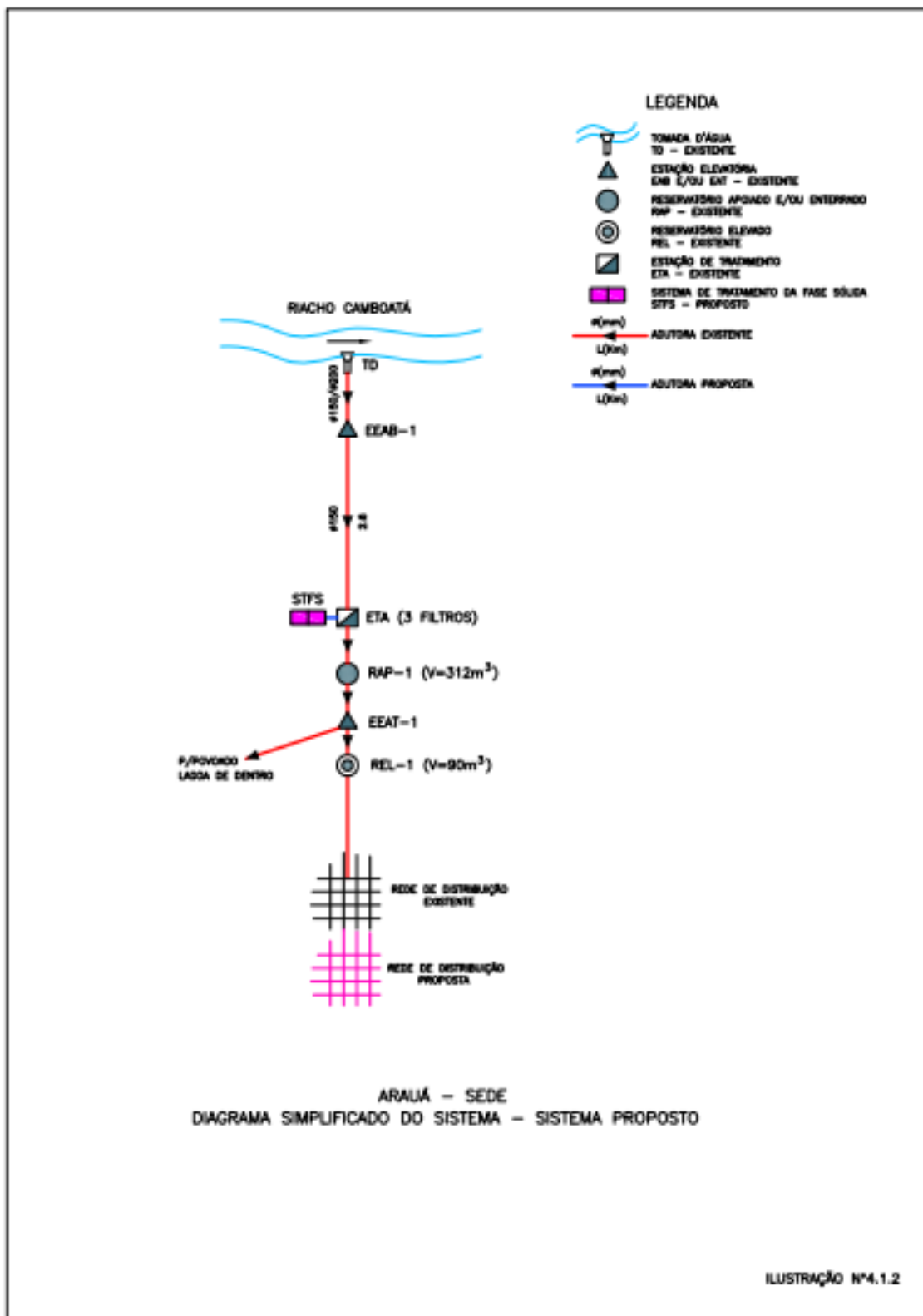
Figura 7 - Sistema Proposto
