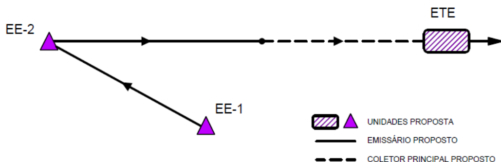
Figura 6 - Sistema de interligação das elevatórias
