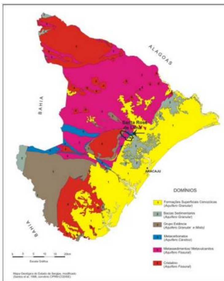
Figura 3 - Domínios Hidrogeológicos do Estado de Sergipe
