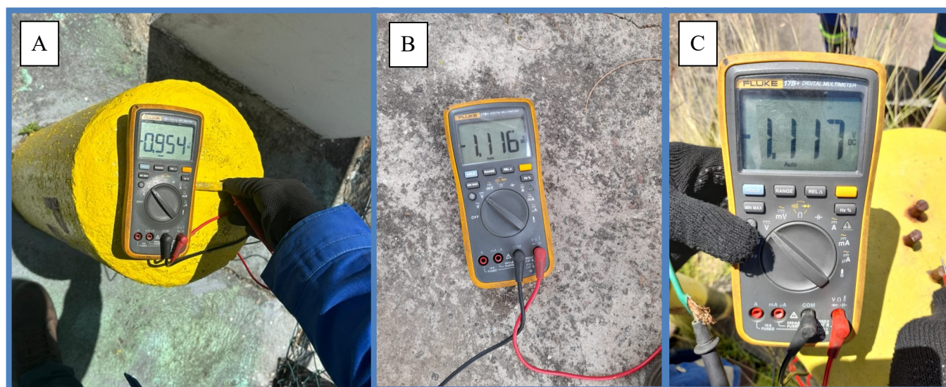
Figura 3: Monitoramento do sistema de proteção catódica por corrente impressa na (A) ETC Estância; (B) ERPM Mosaic e (C) CP-52 Carmópolis.
