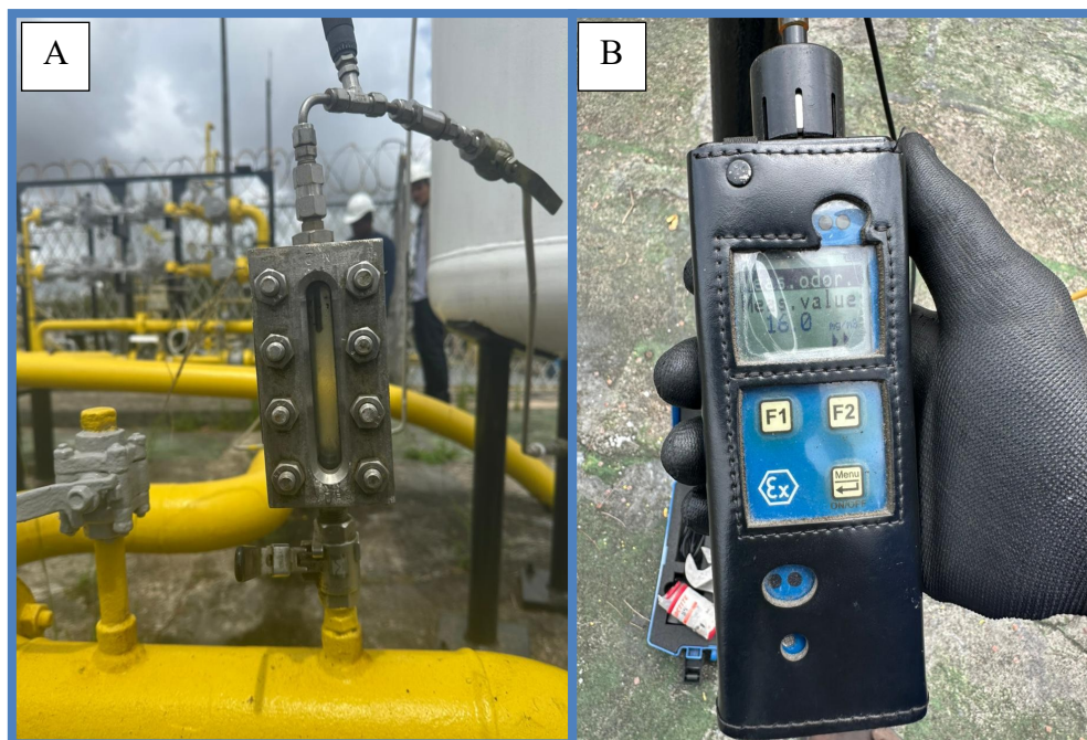
Figura 1: (A) ETC ESTÂNCIA; (B) ERPM AMBEV.
