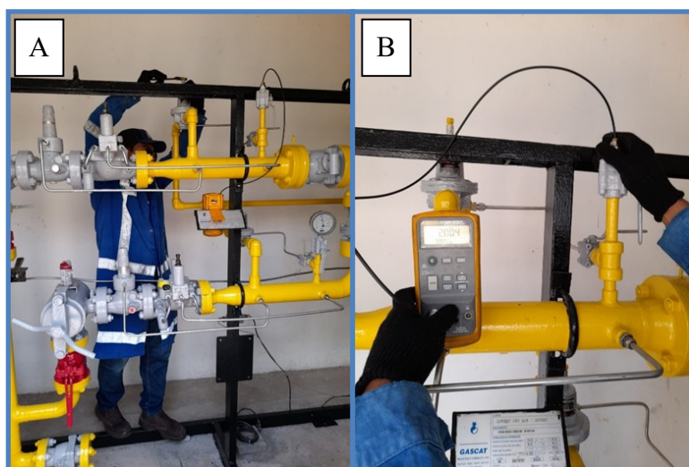
Figura 5 (A e B): Acompanhamento do serviço de ajuste nas válvulas de regulagem e alívio de pressão.
