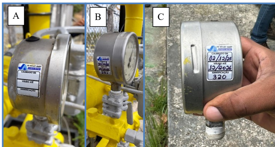
Figura 4 (A, B e C): Acompanhamento do serviço da troca de manômetros.
