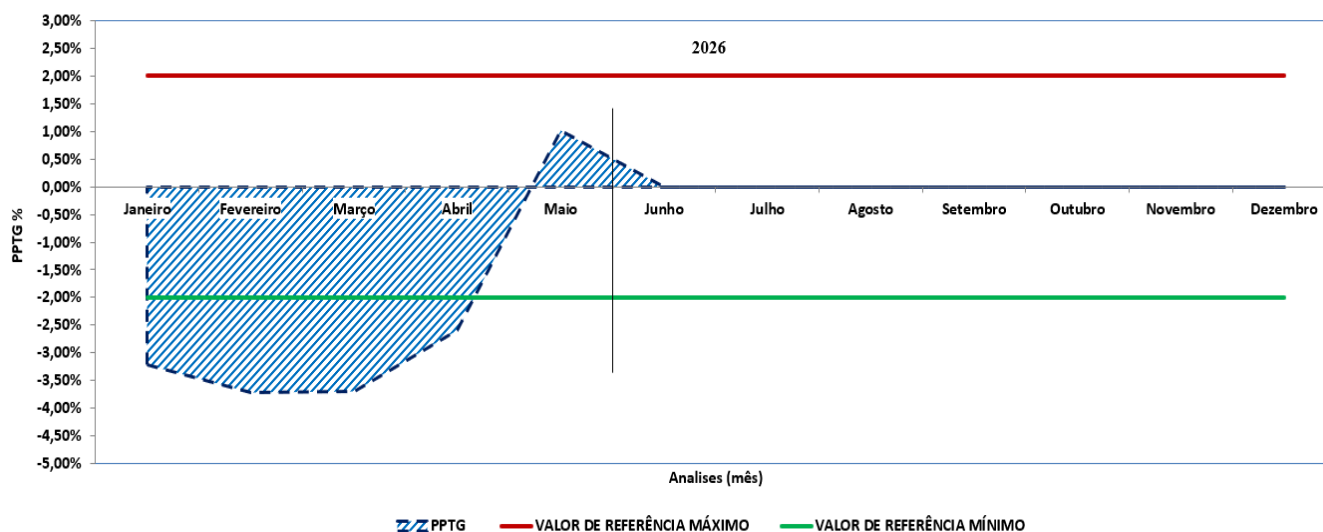
Gráfico 8: Porcentagem de Perdas Totais de Gás: PPTG
