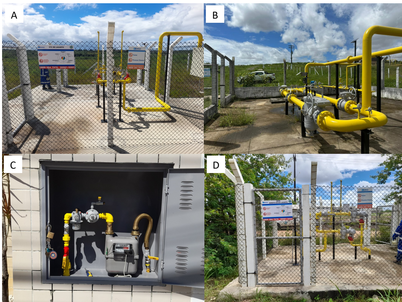
Figura 1: A– ETC Lagarto, B - ETC Socorro, C - CRM do Residencial Saint Sebastian e D - ERPM Maratá Sucos Lagarto.
